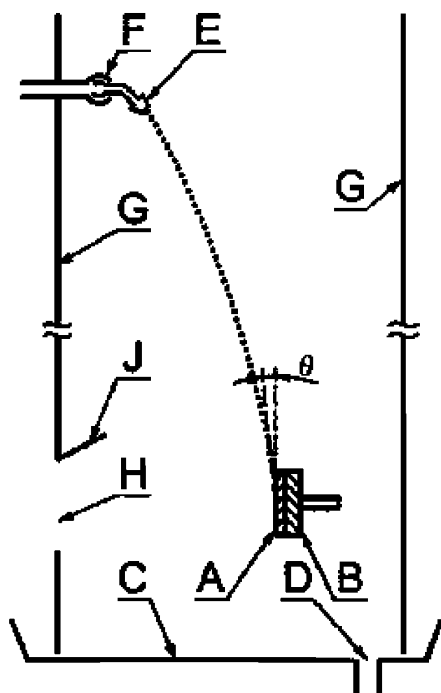
А – проба; В – держатель; С – поддон; D – сточное отверстие; Е – струйное сопло; F – шарнирное соединение; G – корпус; H – квадратное отверстие; J – желоб
